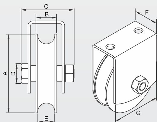
ROLDANA PARA PORTÃO COM BUCHA E PARAFUSO CANAL "U" (Ferro 1/2") C/SUPOORTE
