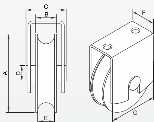
ROLDANA PARA PORTÃO COM PINO CANAL "U" (Ferro 1/2") C/SUPOORTE
